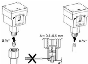
Abb. 3. Druckschalter
