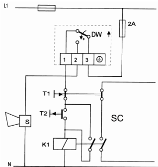
Abb. 6. Maximaldruckbegrenzung
