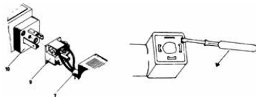
Abb. 2. Verdrahtung
