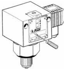
Abb. 10. Mechanische Verriegelung
