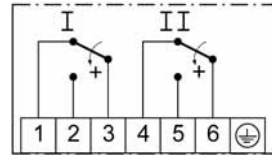
Abb. 13. Anschlußplan
