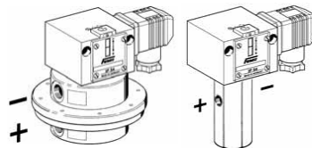
Abb. 4. Druckanschluß
